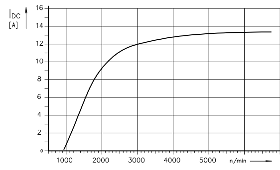
CHARACTERISTIC OF THE SET PROUDOVÁ CHARAKTERISTIKA SOUPRAVY U=14V-konst
