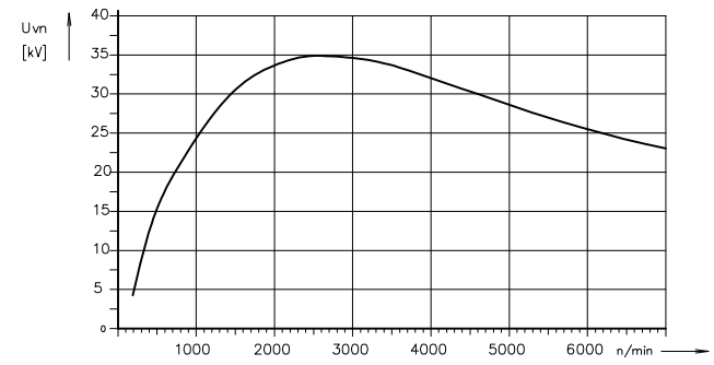
CHARACTERISTIC OF THE HIGH VOLTAGE CHARAKTERISTIKA VYSOKÉHO NAPĚTÍ
